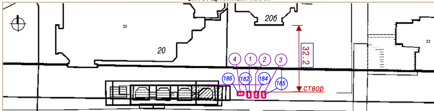
ГРАФИЧЕСКОЕ ИЗОБРАЖЕНИЕ М 1:500 (СХЕМА РАЗМЕЩЕНИЯ НЕСТАЦИОНАРНОГО ТРГОВОГО ОБЪЕКТА)
