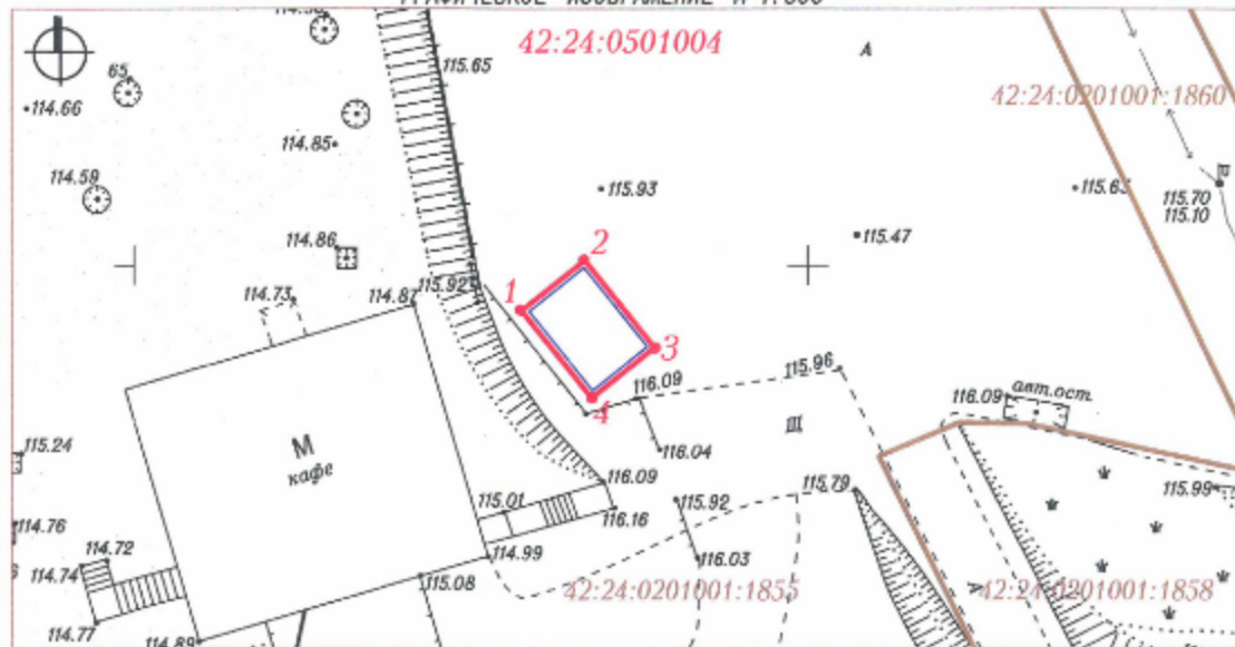
ГРАФИЧЕСКОЕ ИЗОБРАЖЕНИЕ М 1:500
